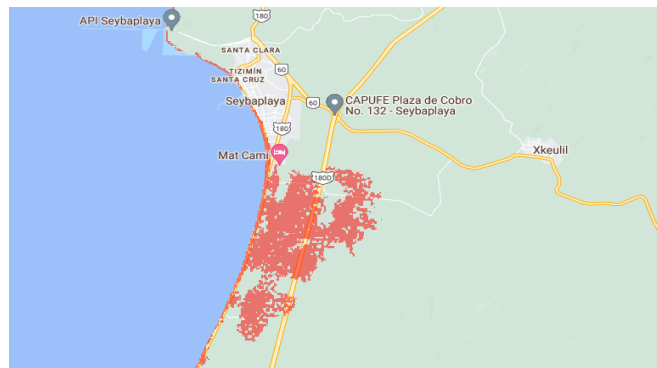
Figura 4.1.4. Áreas inundadas en la cabecera municipal y afectación de las carreteras estatal y federal 180.
